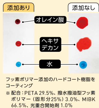
図3 PETフィルムの撥水撥油性
