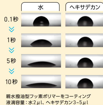
図4 ガラス板に対する接触角比較
