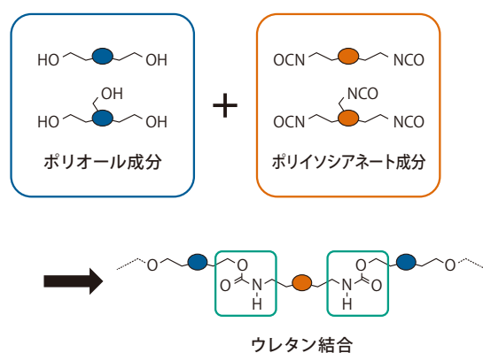
図1 ウレタン反応の概念図
